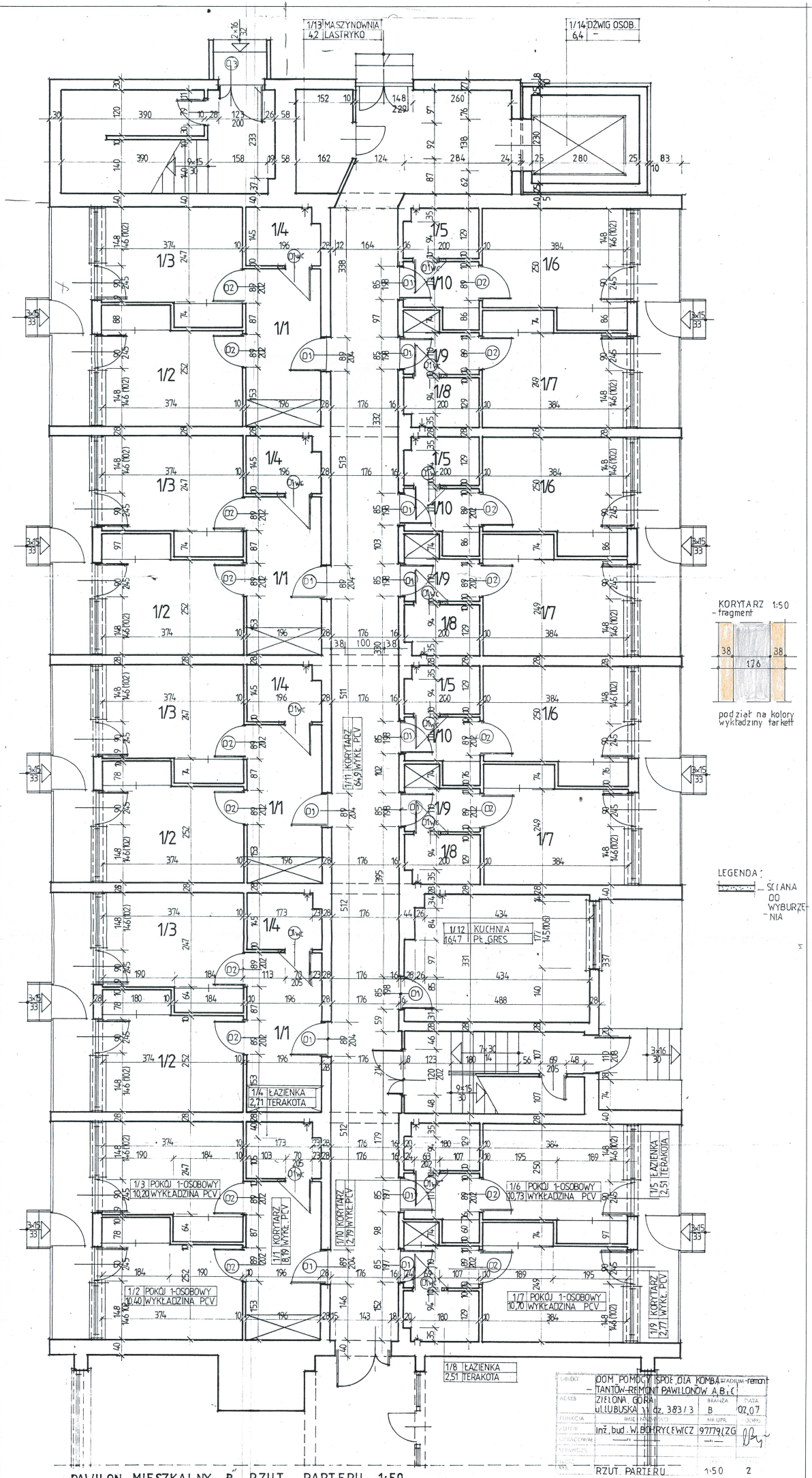
PAWILON MIESZKALNY „B” RZUT PARTERU 1:50 RZUT PARTERU 1:50 2
